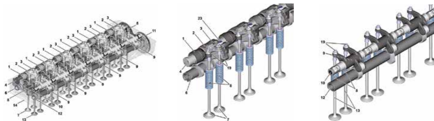
Slika 3: 7-ispušni ventili 12-uisni ventili
