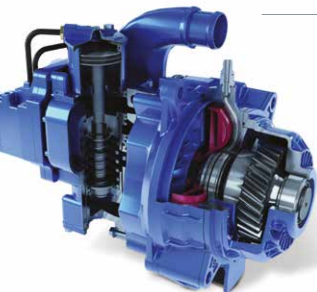
Slika 6: Voith SWR, vodeni retarder
