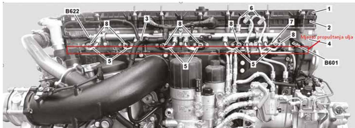
Slika 1. Mjesto propuštanja ulja na vozilu Actros MP4 s motorom OM 470 i OM 471
