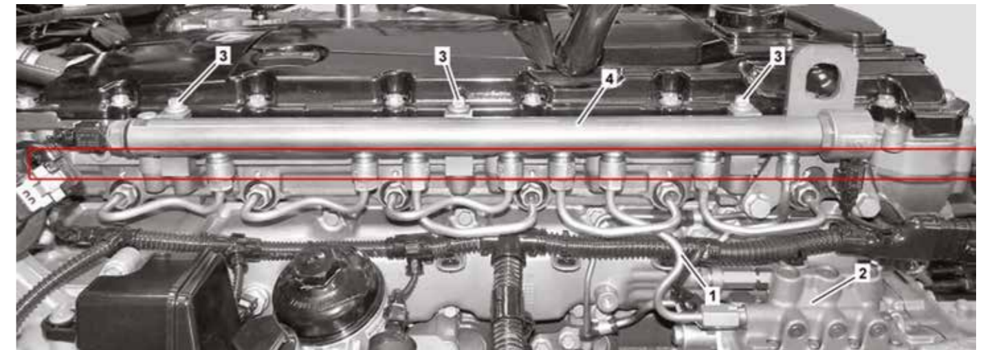
Slika 2. Mjesto propuštanja ulja na vozilu Atego E6 OM 934 i OM 936
